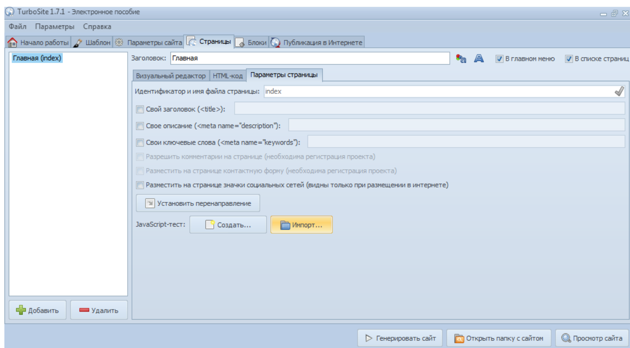
Рис.1.2.9 создание JavaScript-тест
